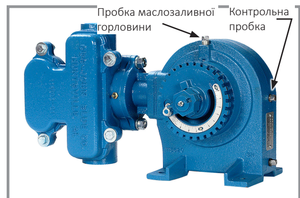
Розташування заливної та контрольної пробки поршневого насоса
