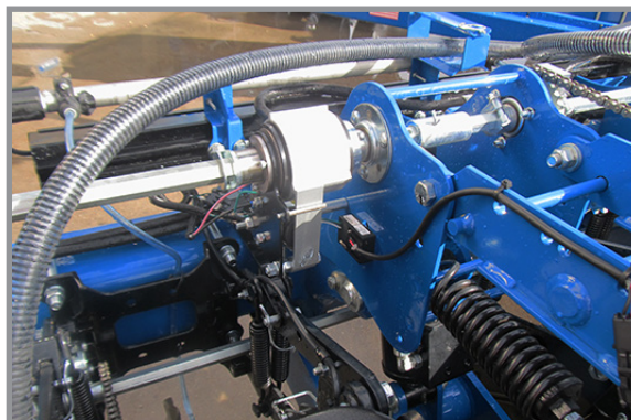
Муфта відключення вказівного ряду
