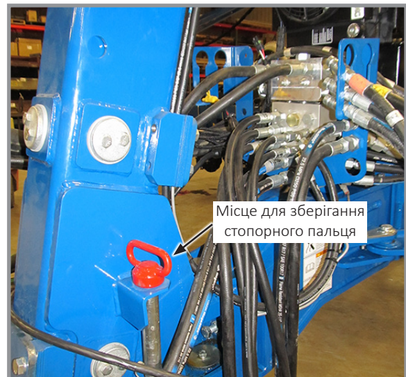
Стопорний палець зчипки дишла
