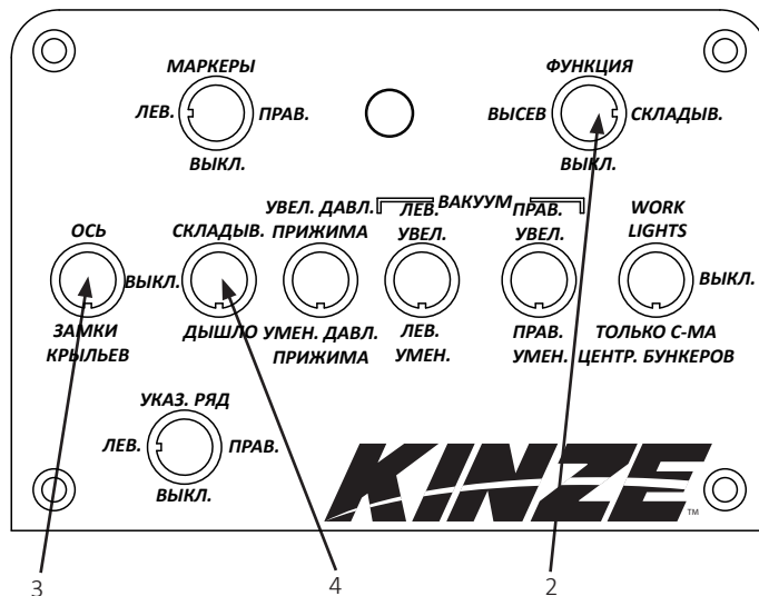
Пульт управления
