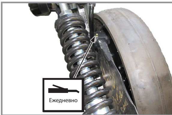
Пресс-масленка — 1 фитинг
