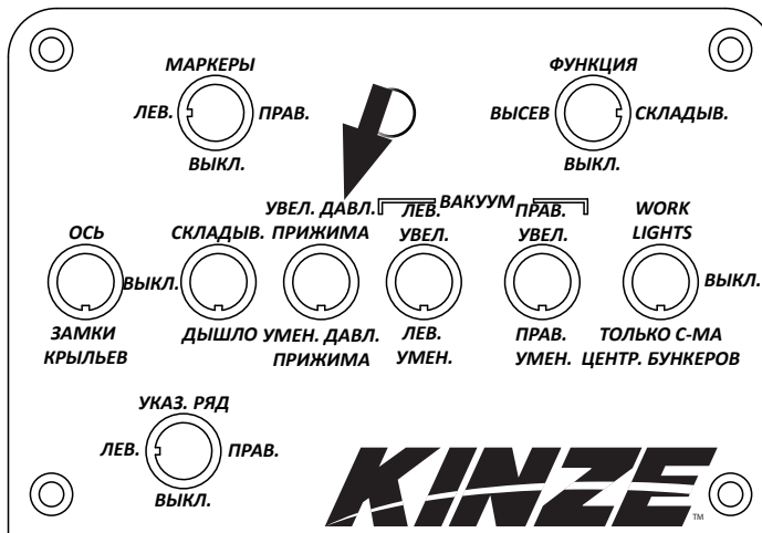
Пульт управления
