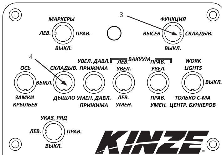
Пульт управления
