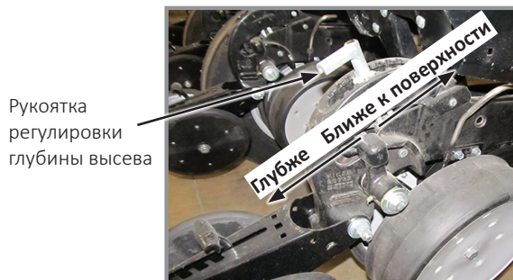
Регулировка глубины высева
