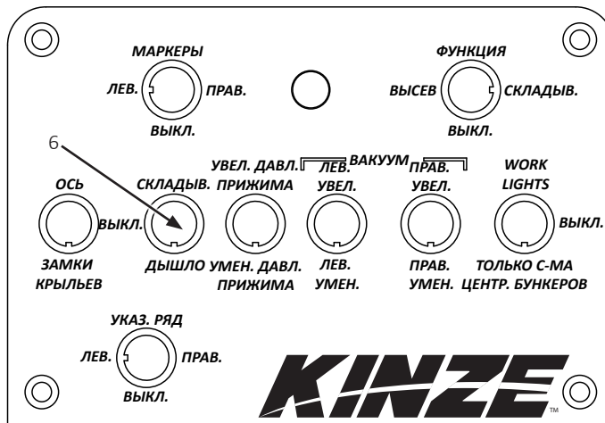
Пульт управления
