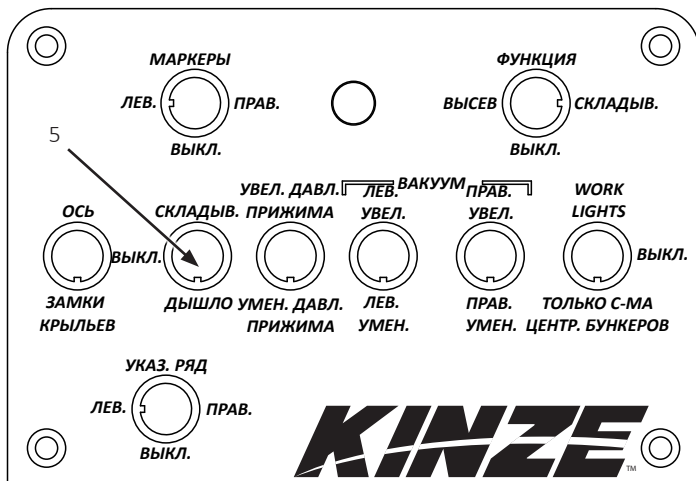
Пульт управления
