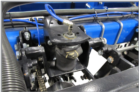
Пневмопружина пружина задней высевающей секции
