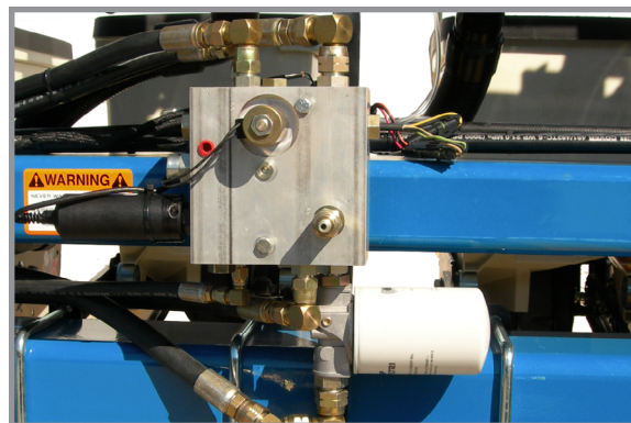
Блок клапанов вакуумного вентилятора
