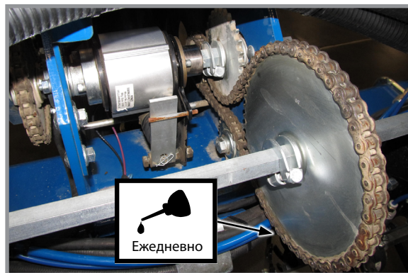
Цепи привода внутреннего модуля (муфта отключения указательного ряда)
