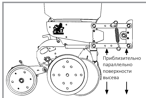
Выравнивание высеваящих секций
