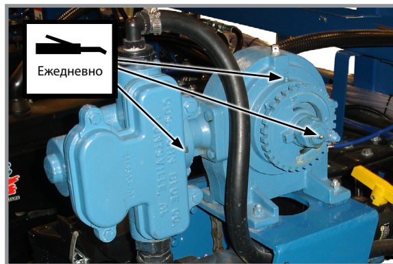
Поршневой насос, правая сторона (3)
