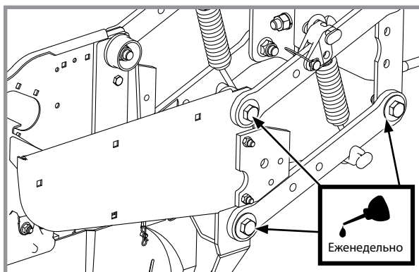
Параллелограммные тяги высевающей секции (по 8 точек смазки на ряд)
