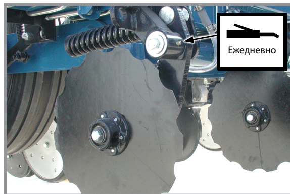
Зубчатый однодисковый сошник (1 на рычаг)
