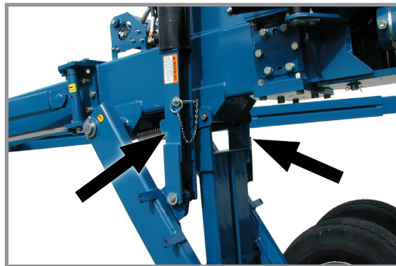
Стопорное устройство в положении для транспортировки/обслуживания
