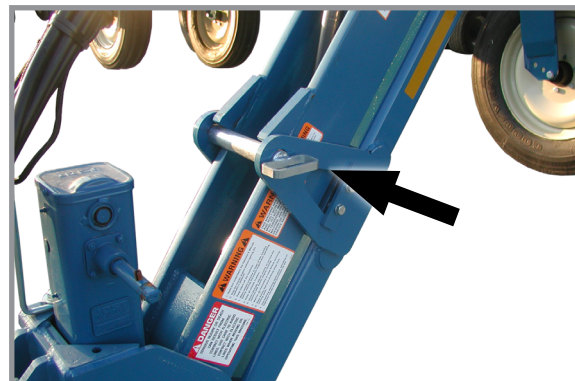
Стопорное устройство параллельных тяг дышла в установленном положении
