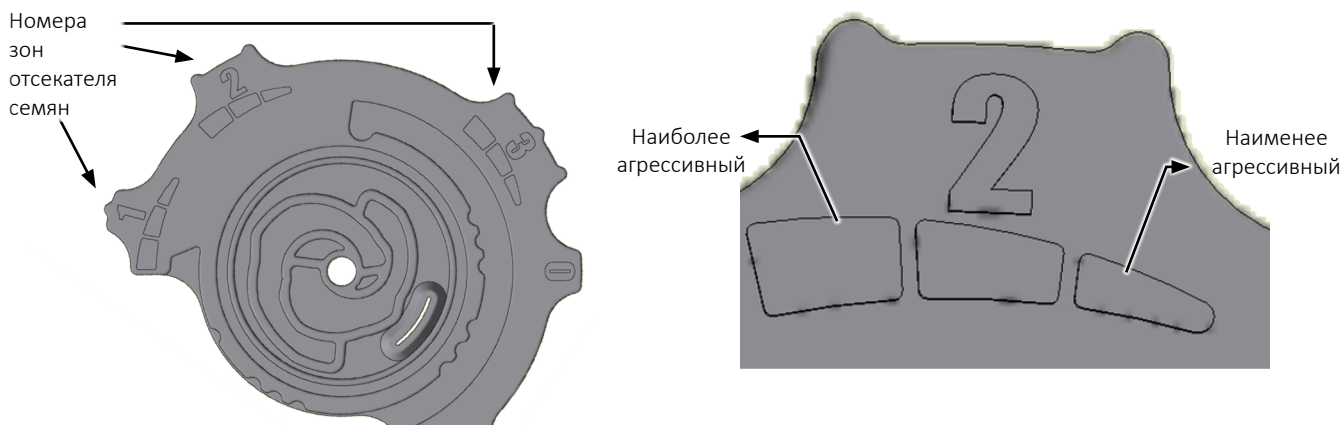
Регулировочное колесо отсекателя семян
