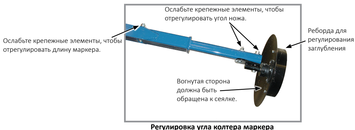
Регулировка угла колтера маркера
