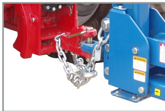
Присоединение предохранительной цепи к трактору
