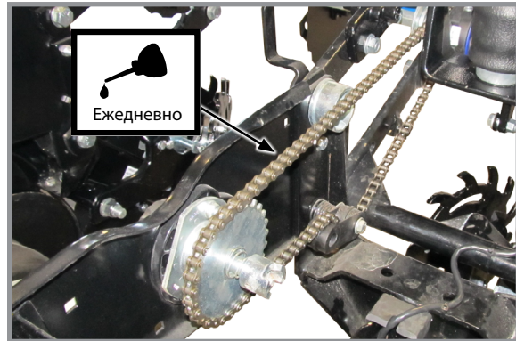
Цепи привода высевающих секций
