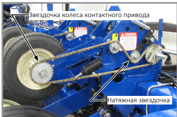
Привод от контактного колеса
