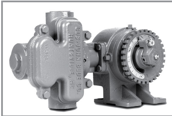
Бутална помпа
