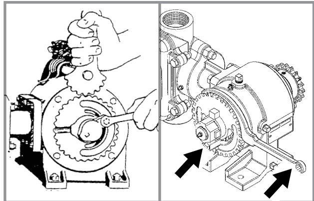
Регулиране на нормата на подаване
