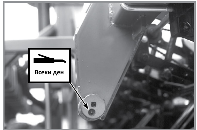
Повдигач със зъбец - 1 на повдигач със зъбец
