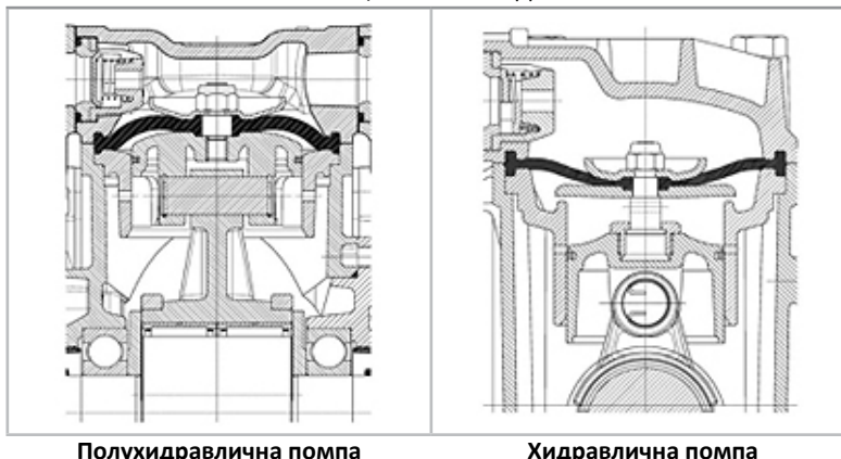
Полухидравлична помпа
