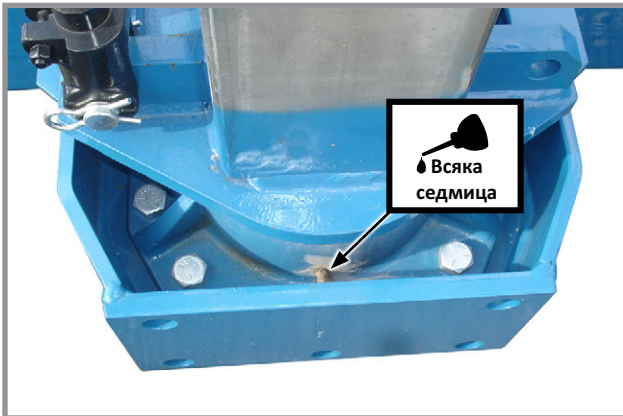
Централна ос - 1
