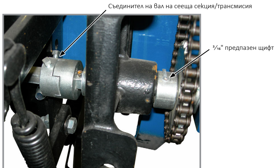
Съединител на вал на трансмисията и вал на сееща секция
