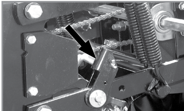
Изключено блокиращо устройство за работа в полеви условия
