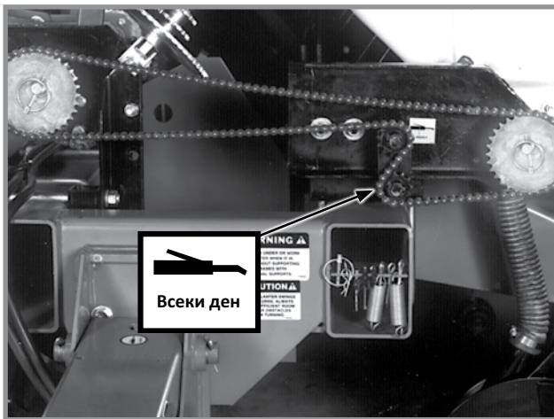
Трансмисия за тор – 1 на трансмисия (натегателна ролка)
