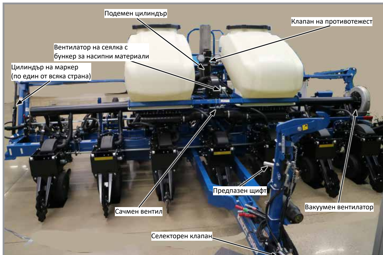
Хидравлична система на модел 3500 (можете да видите схемата в раздел „Смазване и поддръжка“)
