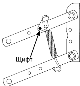
Позиция 1 (най-нисък)
