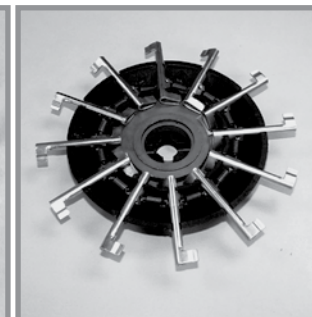
Механизъм с щифтове за маслодаен слънчоглед
