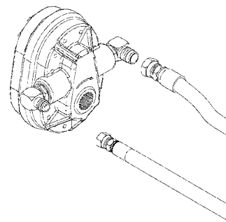
Показана помпа, задвижвана от силоотводен вал, с шлиц 1\frac{3}{8} "-21
