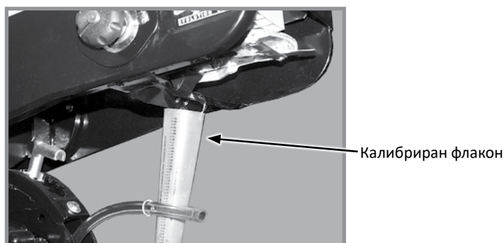
Проверка в работни условия на гранулирани химични препарати
