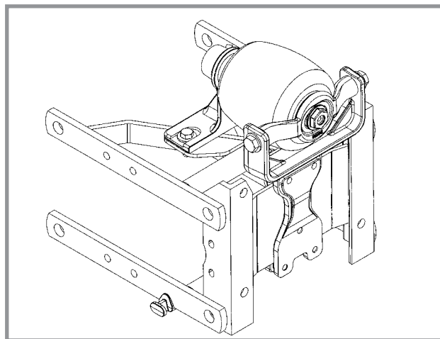
Въздушна пружина на фронтална сееща секция
