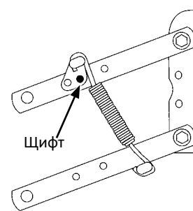
Позиция 4 (най-висок)
