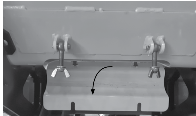
Отворете вратите за почистване на бункера за тор.
