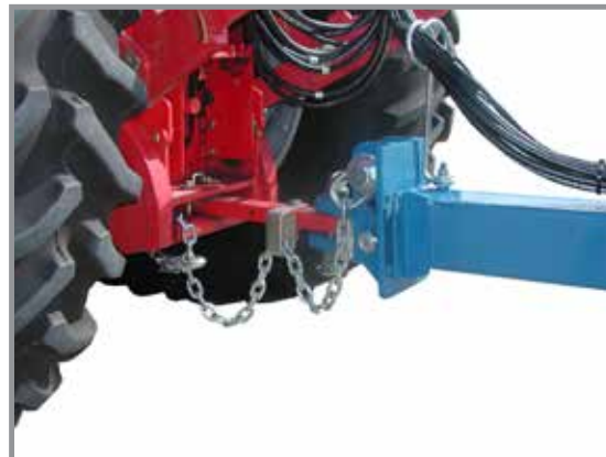
Свързване на теглич и предпазна верига
