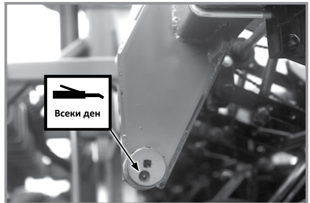
Повдигач със зъбец - 1 на повдигач със зъбец
