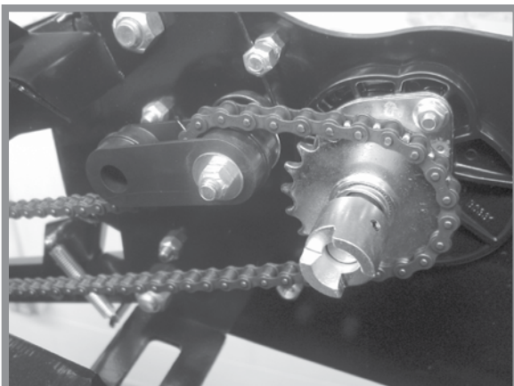
Механичен задвижващ механизъм на изсяващ апарат на фронтална сееща секция
