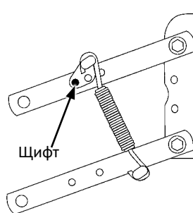
Позиция 3
