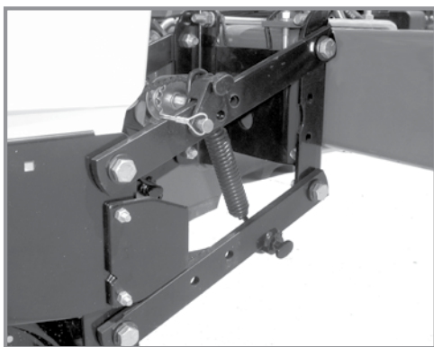
Две пружини на ред (двойни)
