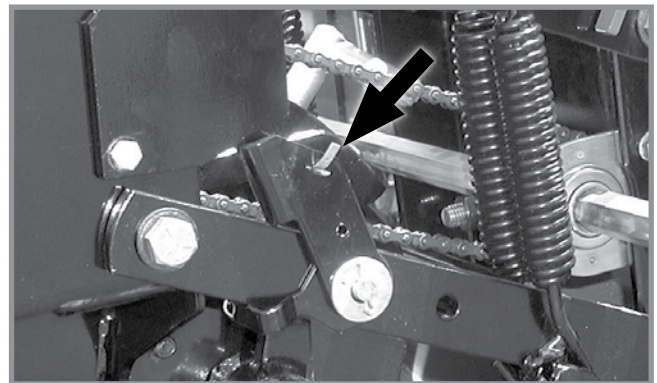
Блокирана фронтална сееща секция в повдигнато положение
