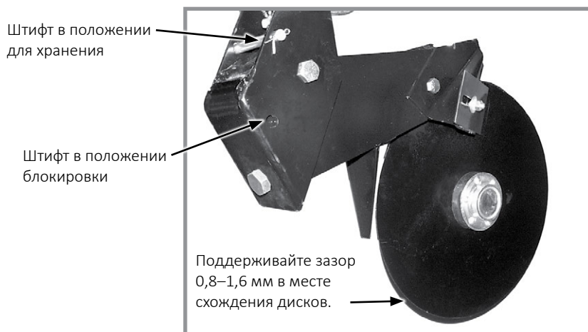
Двухдисковый сошник для внесения удобрений
