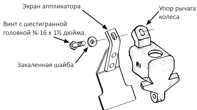
Установка экрана аппликатора для гранулированных удобрений
