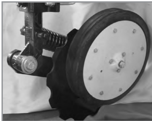
Регулятор заглобления/копирующее колесо зубчатого однодискового сошника
