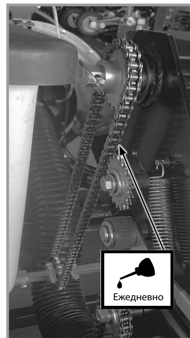
Цепи привода оборудования для внесения сухих удобрений (с обеих сторон узла)
