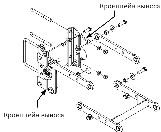
Кронштейны удлинения рычагов секций
