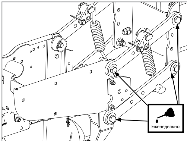
Параллельные тяги крепления задних высевающих секций (по 8 точек смазки на ряд)
