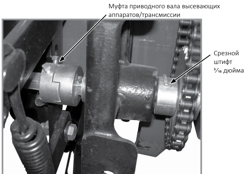
Муфта вала трансмиссии и приводного вала высевающих аппаратов
