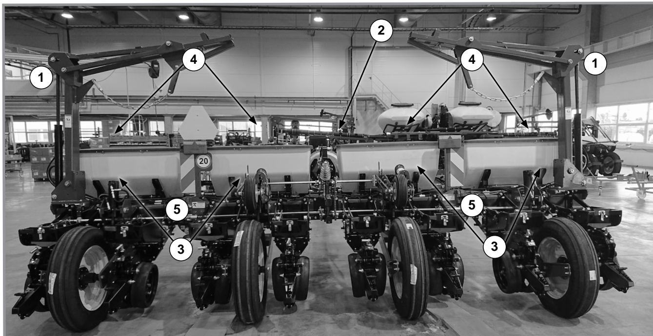
Показана 8-рядная сеялка точного высева модели 3035 с междурядьем 70 см
