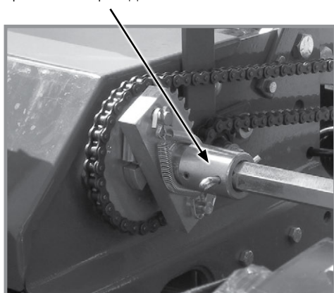
Привод системы внесения жидких удобрений
