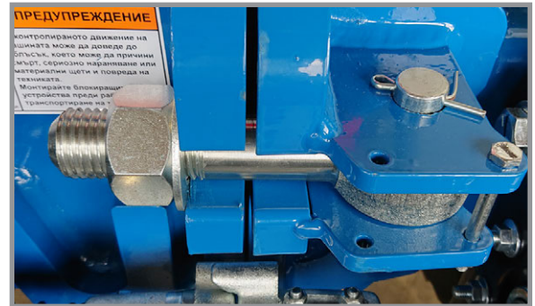
Затяжка фиксирующего крыло болта с кольцом
