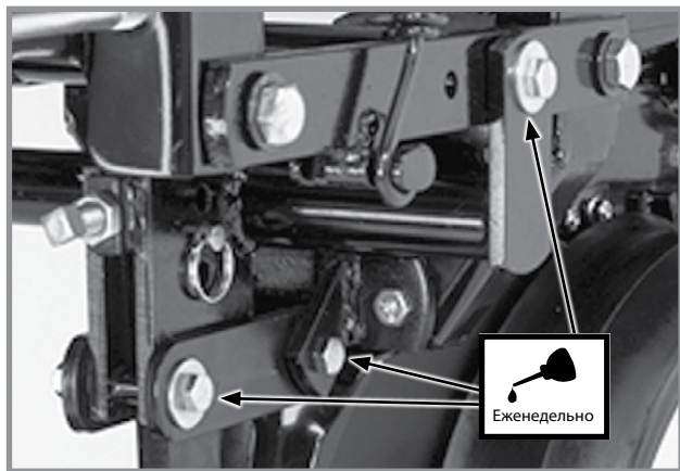
Параллелограммное навесное устройство дискового борозделателя с креплением на высевающей секции (по 6 точек смазки на ряд)
