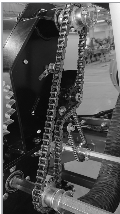
Привод системы внесения сухих удобрений
