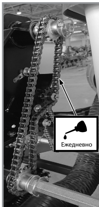
Цепи привода оборудования для внесения сухих удобрений (с обеих сторон узла)
