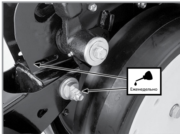
Эксцентриковые втулки (по 2 точки смазки на ряд) V-образного заделывающего колеса и/или прицепного заделывающего колеса высевающей секции.
