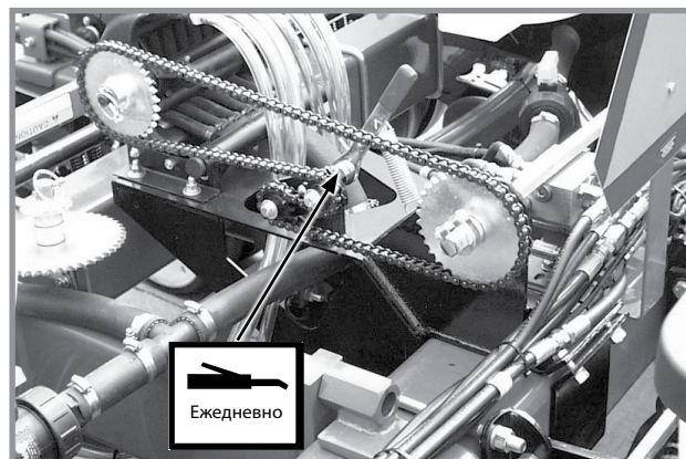
Натяжитель цепи привода поршневого насоса — 1
