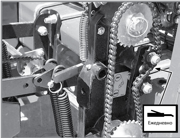
2. Трансмиссия нормы высева — 1 точка смазки (натяжитель)
