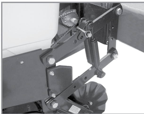
Четыре пружины на ряд (только дисковые ножи для нулевой обработки почвы, устанавливаемые на высевающие секции)
