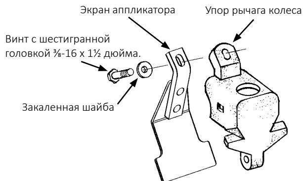
Установка экрана аппликатора для гранулированных удобрений
