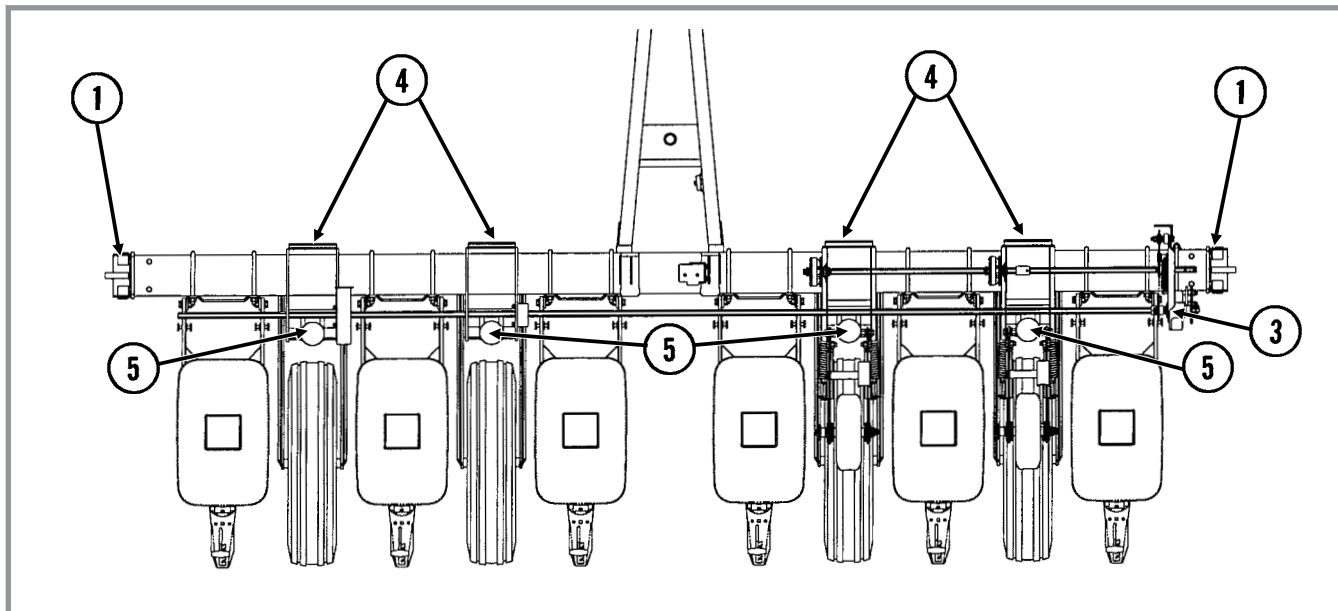
Показана 6-рядная селка точного высева модели 3000 с междурядьем 70 см
