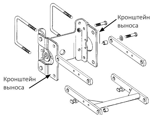
Кронштейны удлинения рычагов секций
