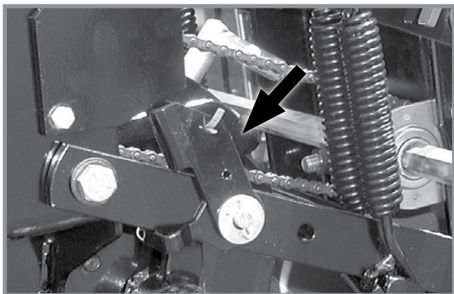
Фронтальная высевающая секция, заблокированная в поднятом положении
