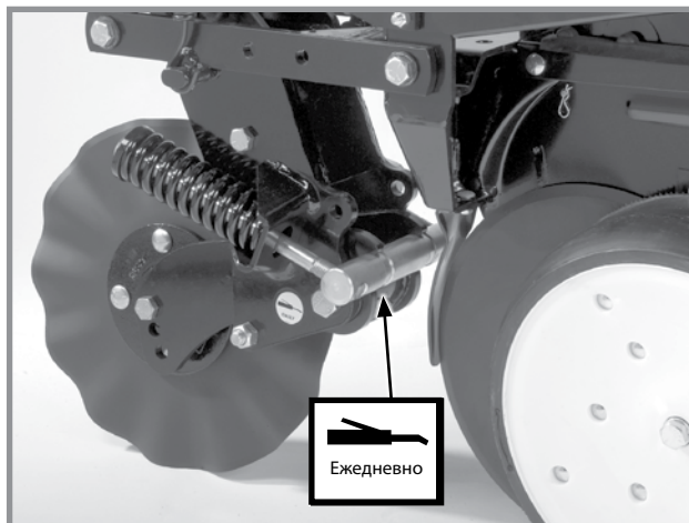
Дисковый нож с креплением на раме — по 1 на рычаг
