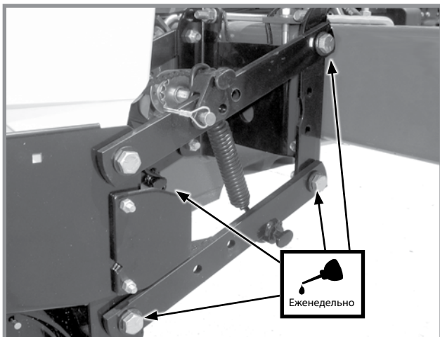
Параллельные тяги крепления задних и/или фронтальных высевающих секций (по 8 точек смазки на ряд)
