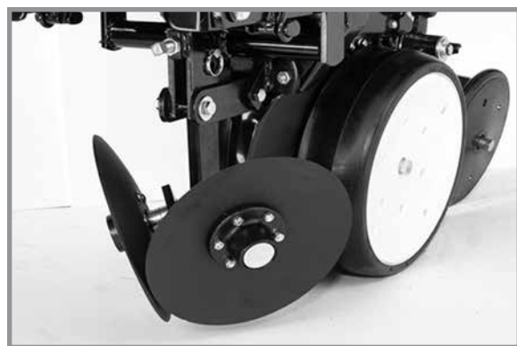
Дисковый бороздоделатель с креплением на высевающей секции
