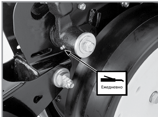
Рычаги копирующих колес — по 1 на рычаг (Уплотнения в рычагах установлены таким образом, что их кромка направлена наружу, что позволяет смазке вытеснять загрязнения из уплотнения. Закачивайте смазку в рычаг, пока свежая смазка не выступит между шайбами и рычагом.)
